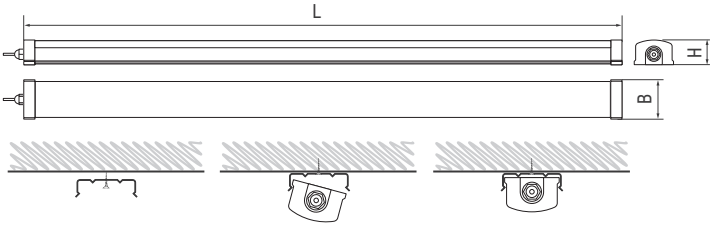
Рис.2 Схема монтажа светильника
